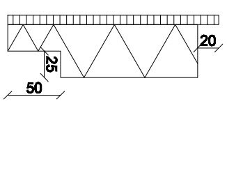
Doorsnede B-B, schaal 1:5
