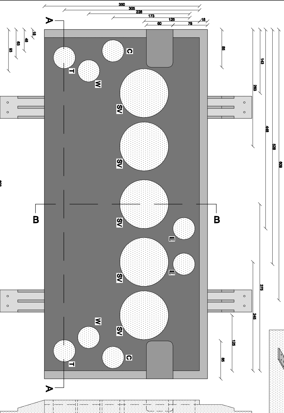
doorsnede B-B, schaal 1:5
