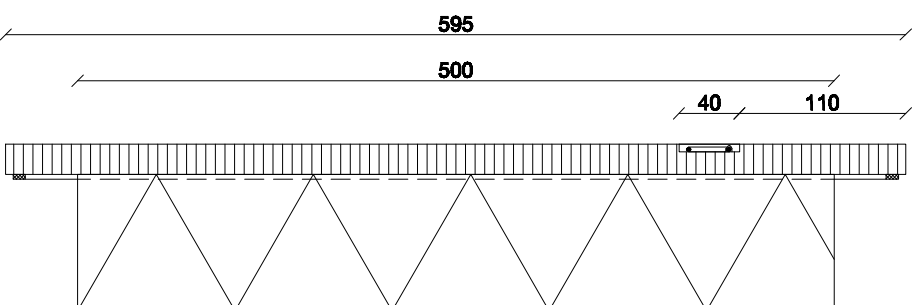
Doorsnede B-B
